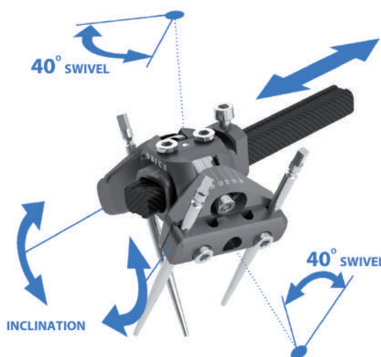
Esempio: Adattatore Barra-Morsetto Rotante con due Base-Morsetto Rotanti e con disposizione a V delle fiches
